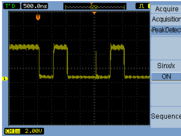
图 32 峰值检测波形
