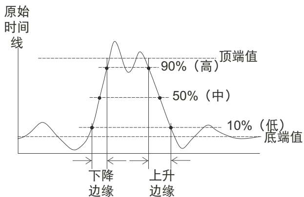
图 41 上升时间和下降时间测量
