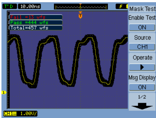
图 53 通过测试显示
