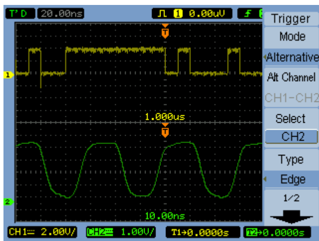
图 36 交替触发
