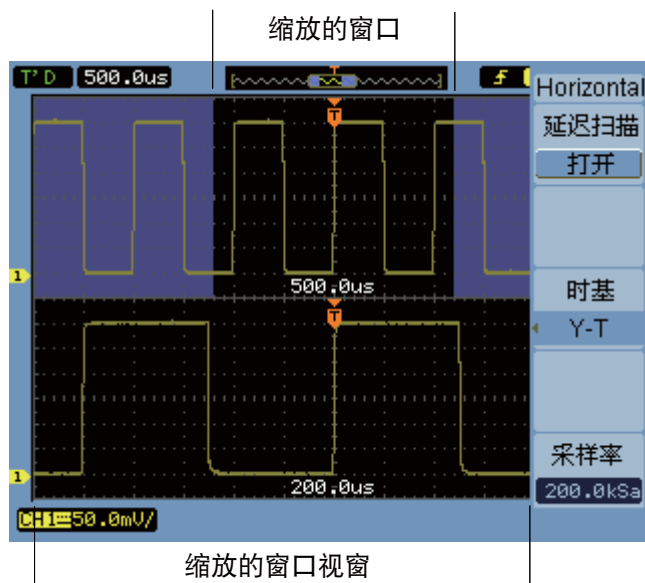
图 13 缩放的时基窗口
