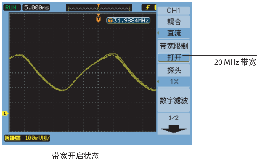
图 19 带宽限制控件打开
