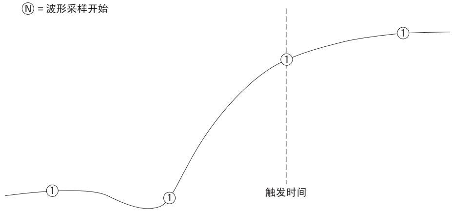
图 28 实时采样模式
