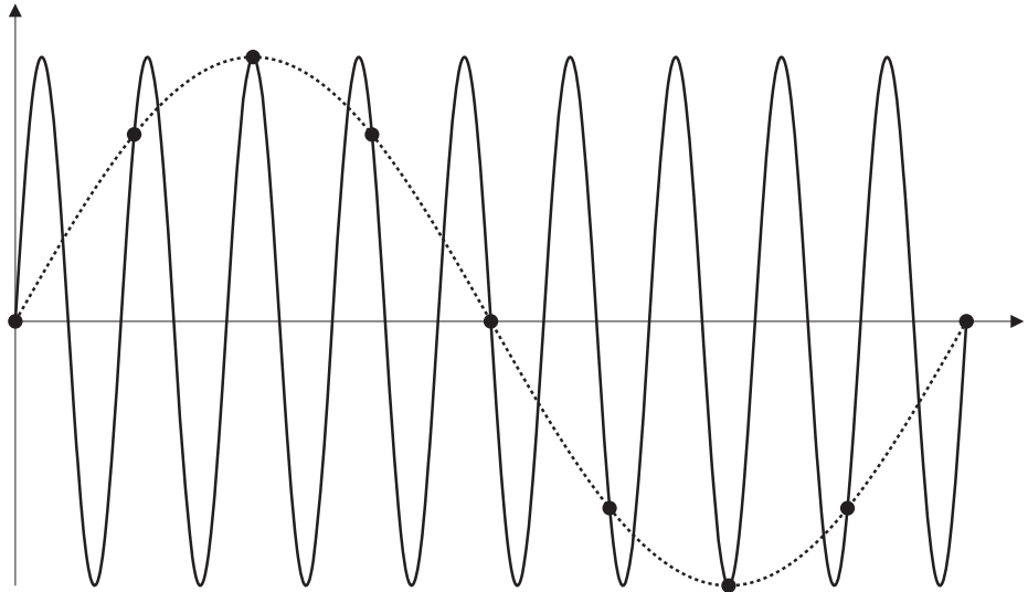
图 25 混叠
