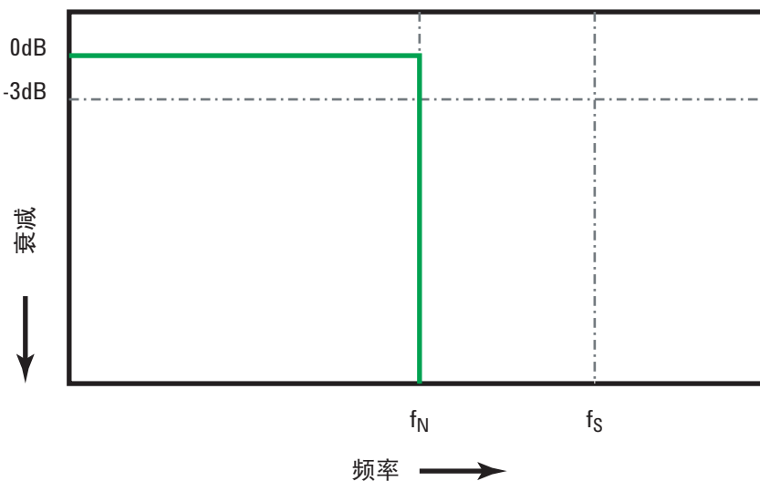
图 26 理论砖墙频率响应
