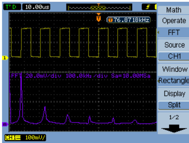
图 23 FFT 波形
