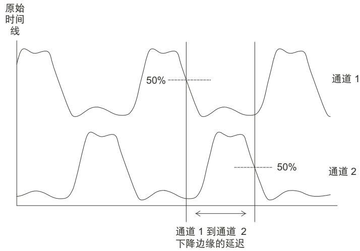
图 43 延迟测量
