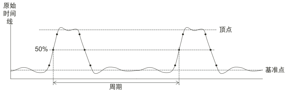
图 40 周期和频率测量
