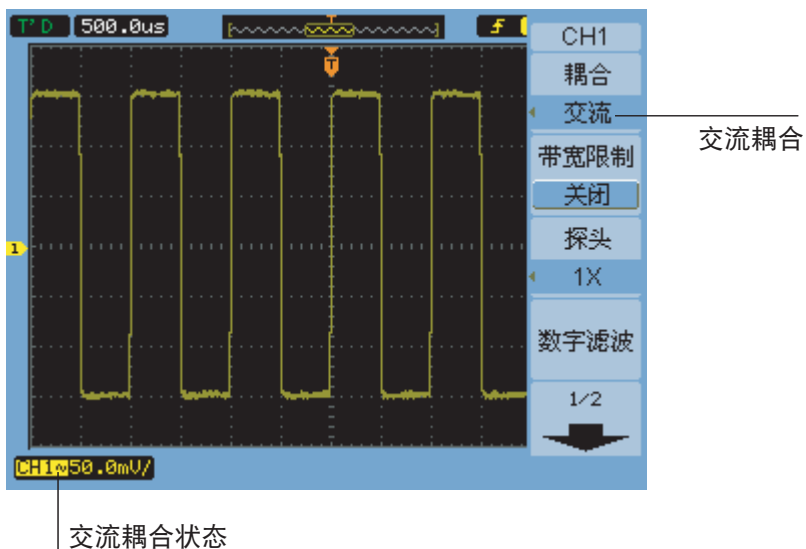
图 17 交流耦合控件
