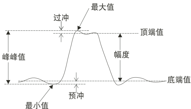
图 39 电压测量点
