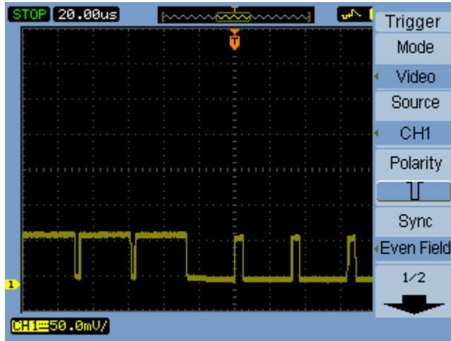
图 35 场同步
