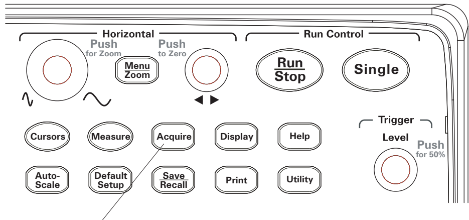
图 29 采集 [Acquire] 键
