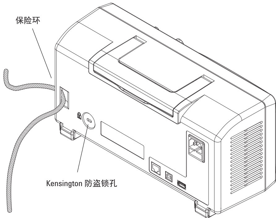
图 10 固定仪器
