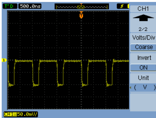
图 21 反相后的波形
