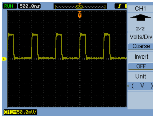
图 20 反相前的波形
