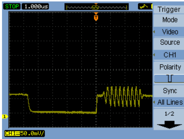
图 34 行同步
