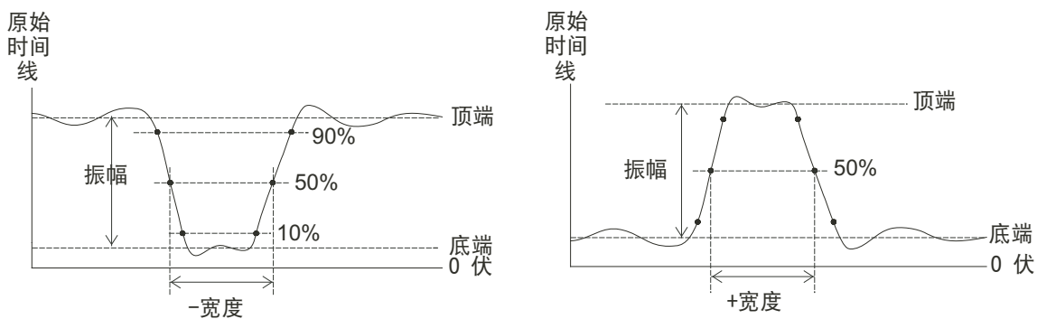
图 42 正脉冲宽度和负脉冲宽度测量
