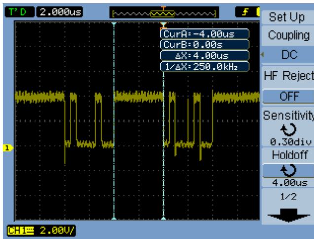
图 37 触发释抑
