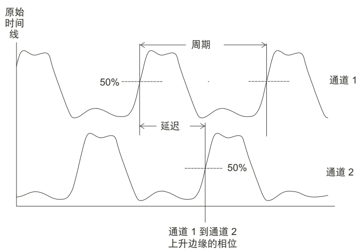
图 44 相位测量
