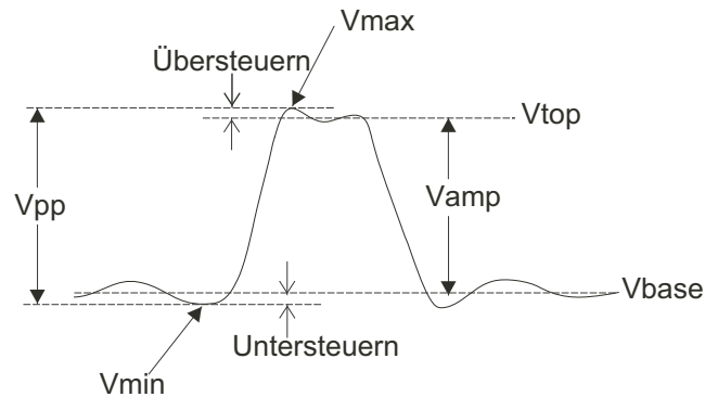
Abbildung 39 Referenzpunkte für Spannungsmessungen
