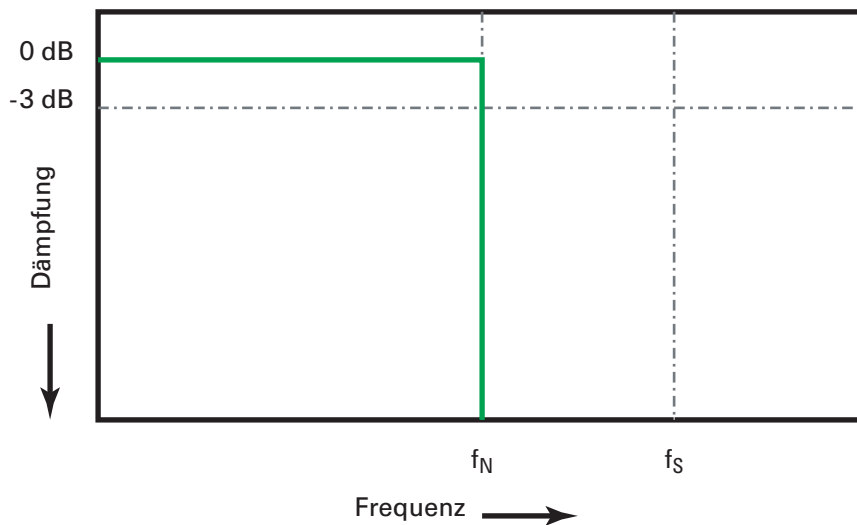
Abbildung 26 Theoretische „Brick-Wall“ Frequenzreaktion
