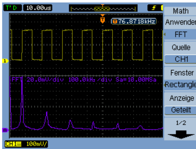
Abbildung 23 FFT-Kurve
