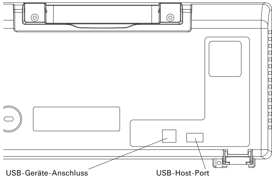
Abbildung 50 USB-Anschlüsse auf der Rückabdeckung
