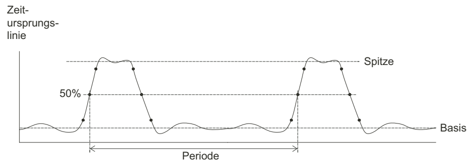
Abbildung 40 Perioden und Frequenzmessungen
