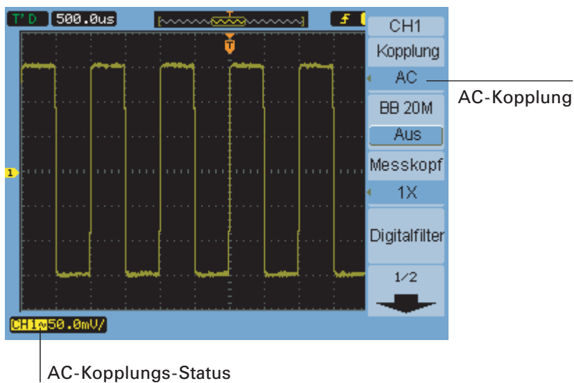
Abbildung 17 AC-Kopplungseinstellung
