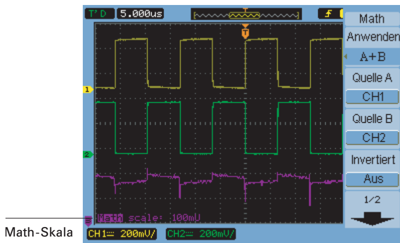
Abbildung 22 Einstellungswerte für mathematische Funktionen
