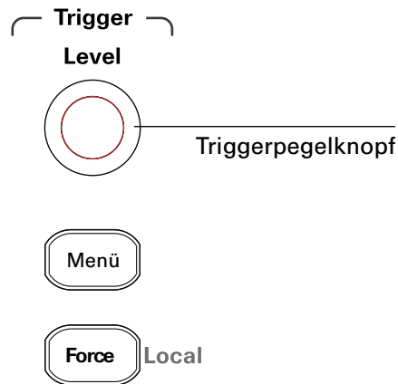
Abbildung 33 Trigger-Einstellungen
