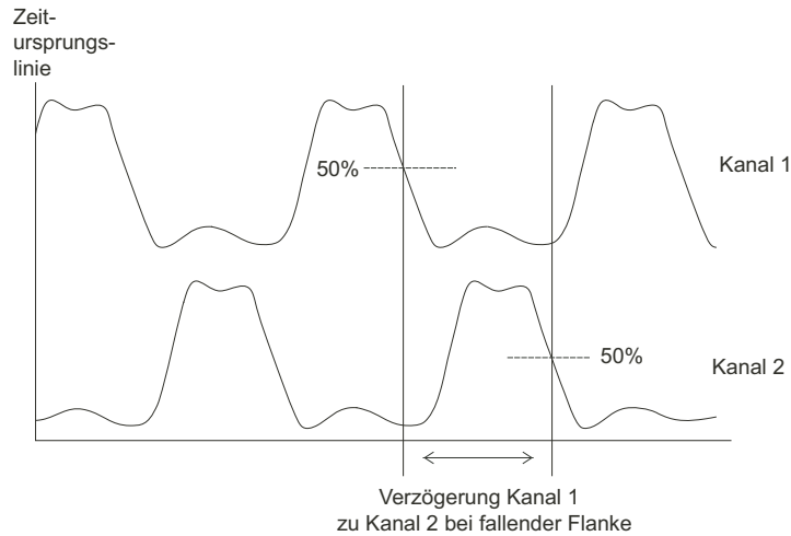
Abbildung 43 Verzögerungsmessung
