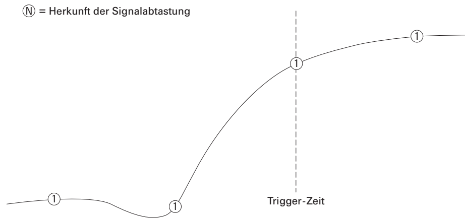
Abbildung 28 Echtzeitabtastmodus
