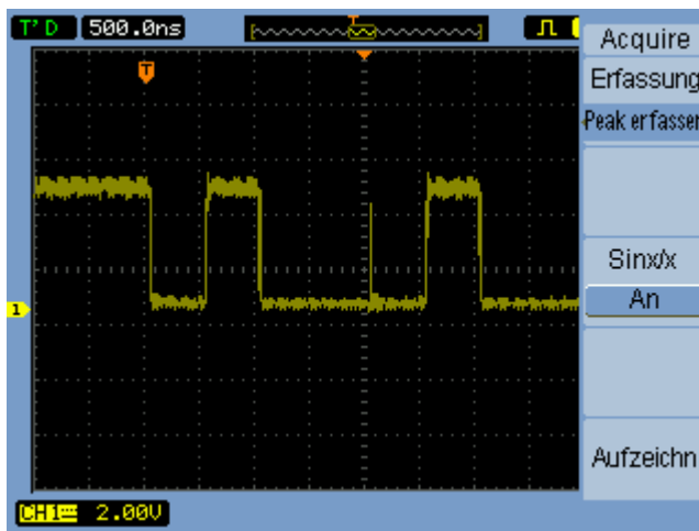
Abbildung 32 Mit dem Modus Peak erfassen erfasstes Signal
