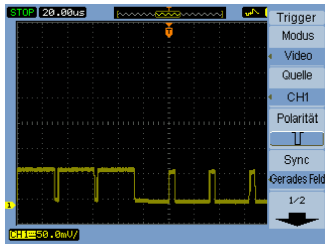
Abbildung 35 Feldsynchronisation
