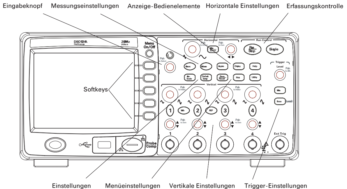
Abbildung 5 Frontabdeckung
