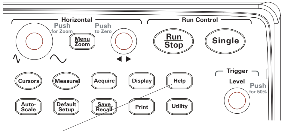
Abbildung 9 Taste Hilfe [Help]
