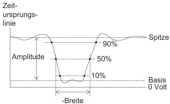
Abbildung 42 Messung der positiven und negativen Impulsbreiten
