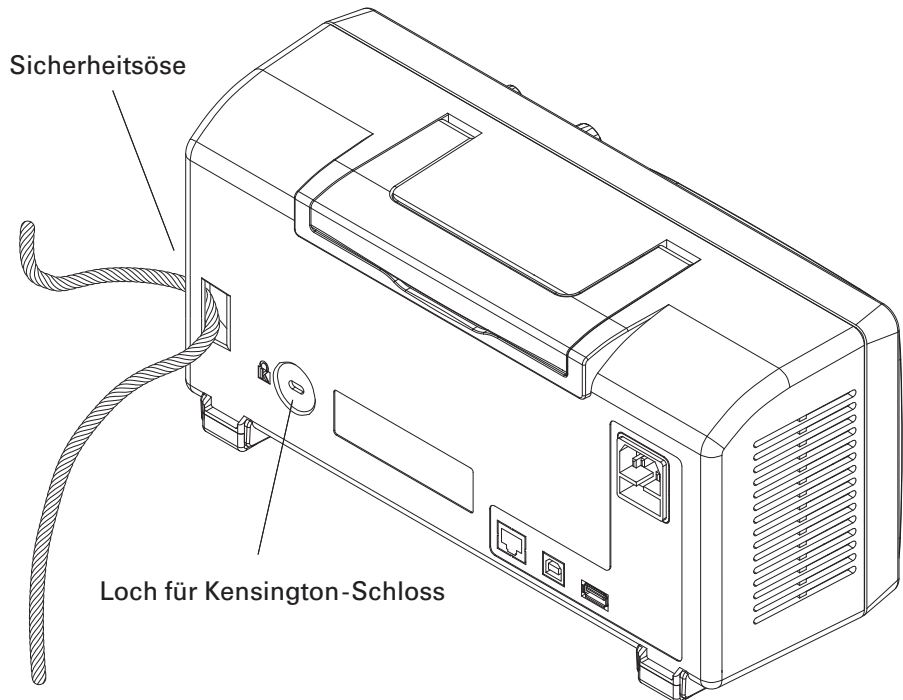
Abbildung 10 Gerät sichern
