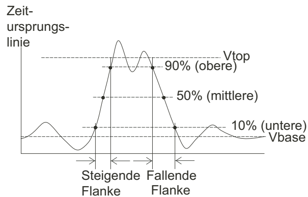
Abbildung 41 Messung der Anstiegs- und Abfallzeiten
