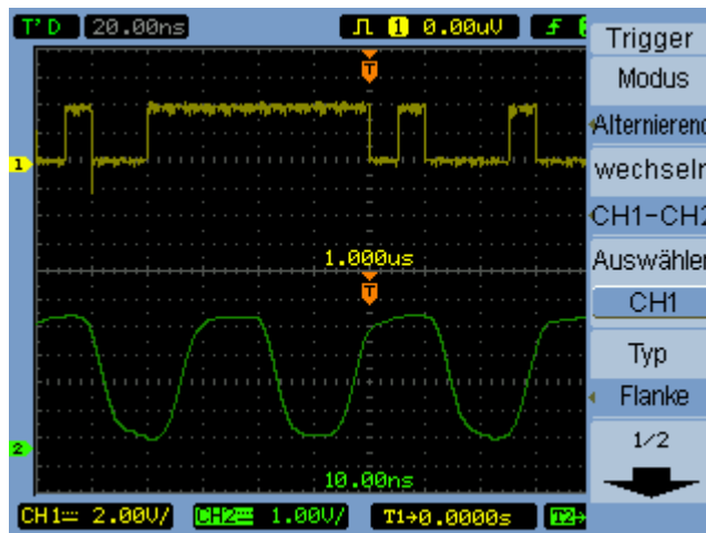
Abbildung 36 Alternierende Triggerung
