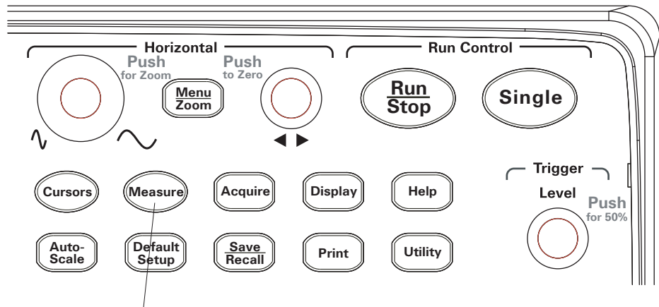
Abbildung 38 Taste Messungen [Measure]
