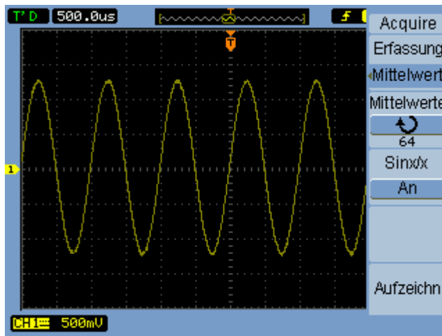
Abbildung 31 Verrauschtes Signal mit Mittelwertbildung
