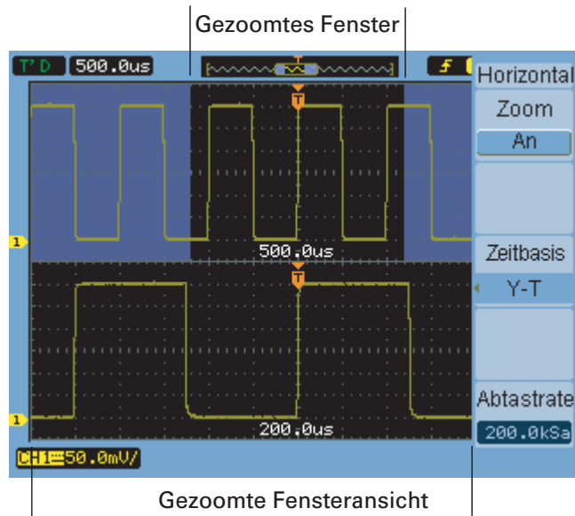
Abbildung 13 Fenster Gezoomte Zeitbasis
