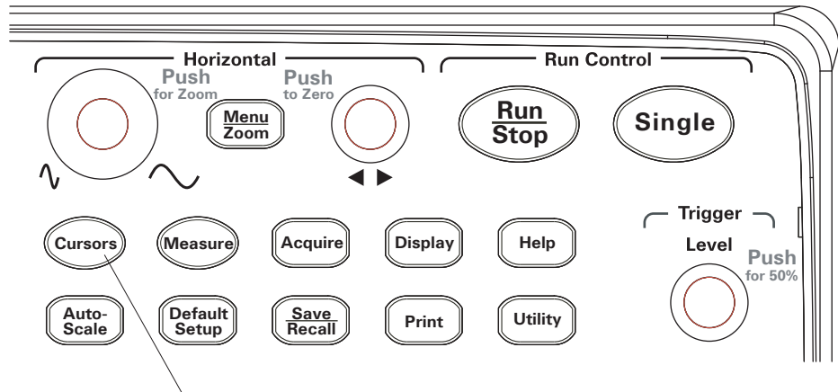
Abbildung 45 Taste Cursor [Cursors]
