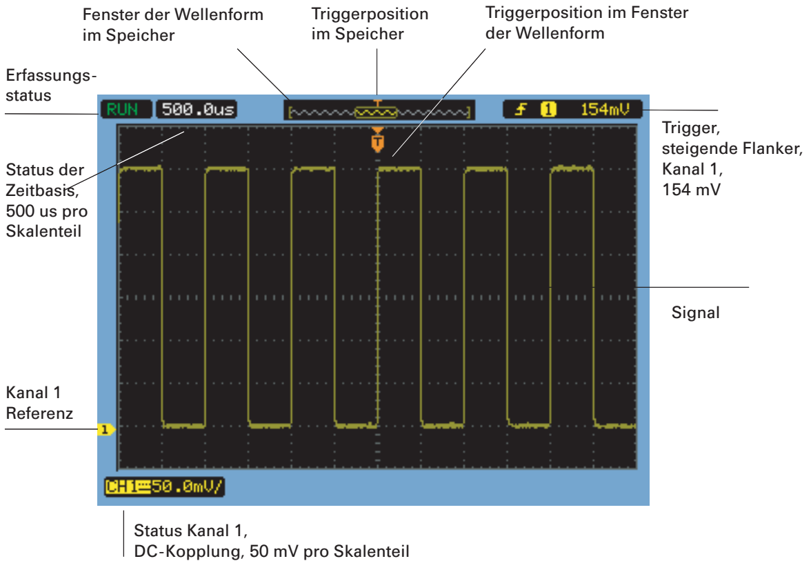
Abbildung 7 Oszilloskopanzeige
