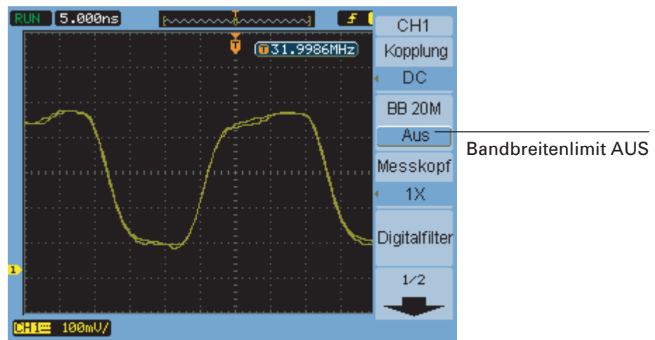
Abbildung 18 Bandbreitenlimit-Einstellung AUS
