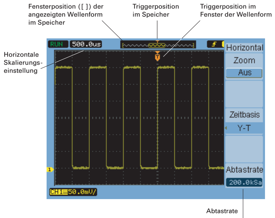
Abbildung 12 Statusleiste, Anzeige der Triggerposition und der horizontalen Skalierung
