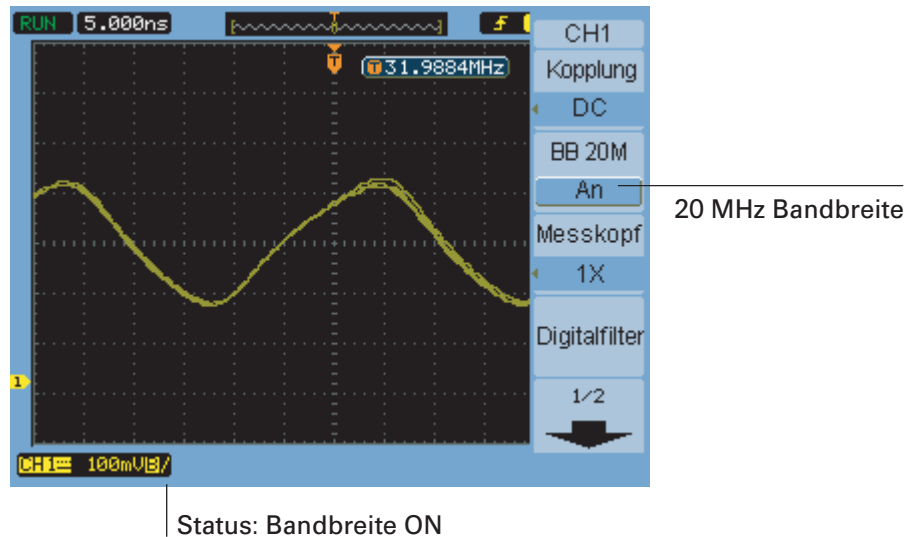
Abbildung 19 Bandbreitenlimit-Einstellung AN
