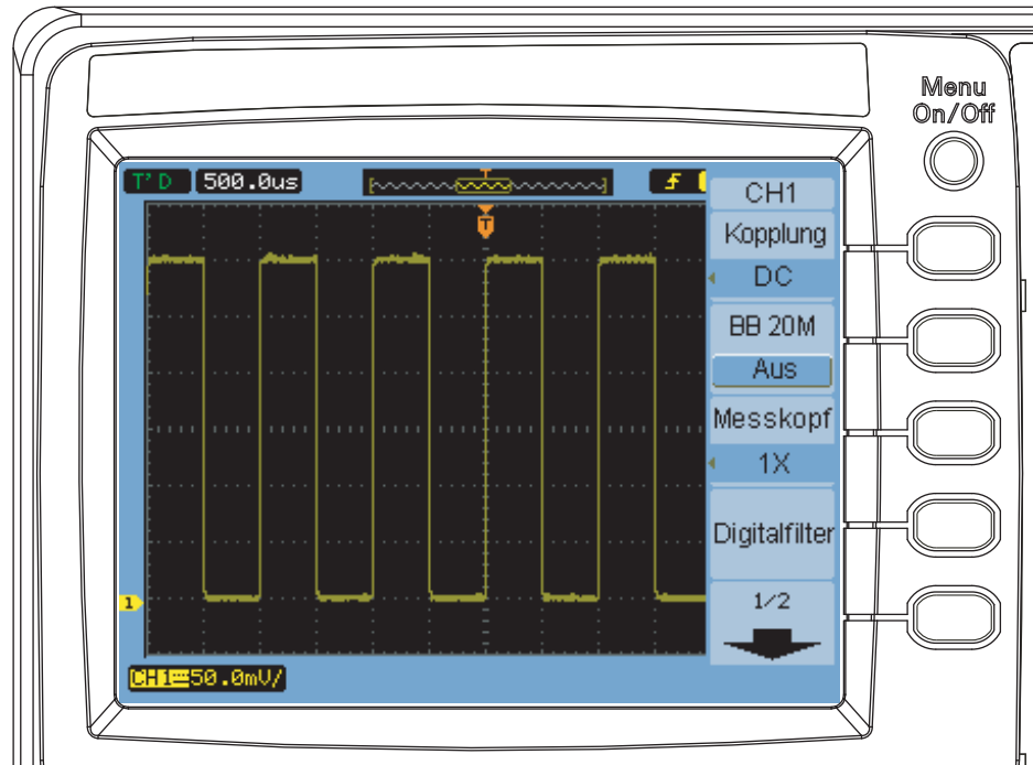
Abbildung 6 Softkey-Menüs
