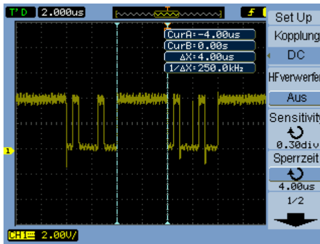
Abbildung 37 Triggerverzögerung
