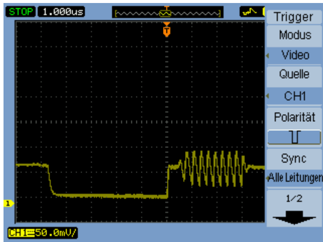
Abbildung 34 Leitungssynchronisation
