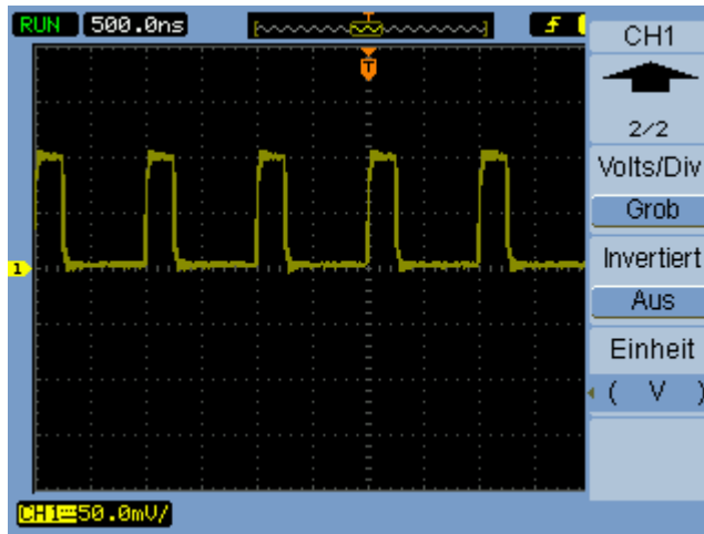
Abbildung 20 Signal vor der Invertierung
