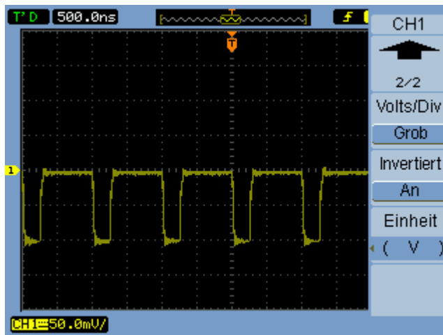
Abbildung 21 Signal nach der Invertierung
