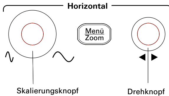
Abbildung 11 Horizontal-Bedienelemente
