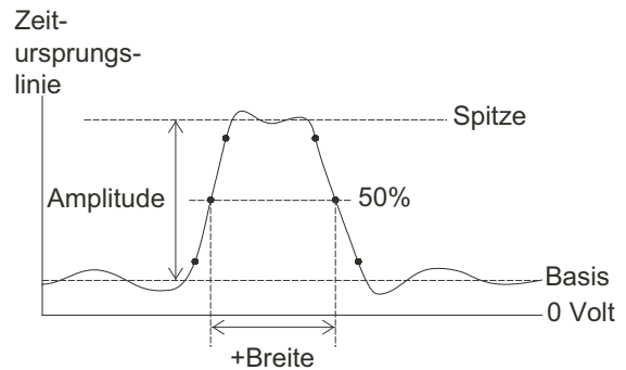
Abbildung 42 Messung der positiven und negativen Impulsbreiten
